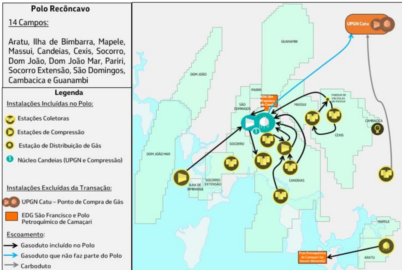
Figura 1 - Fluxo da Produção de Gás Natural do Polo Recôncavo
