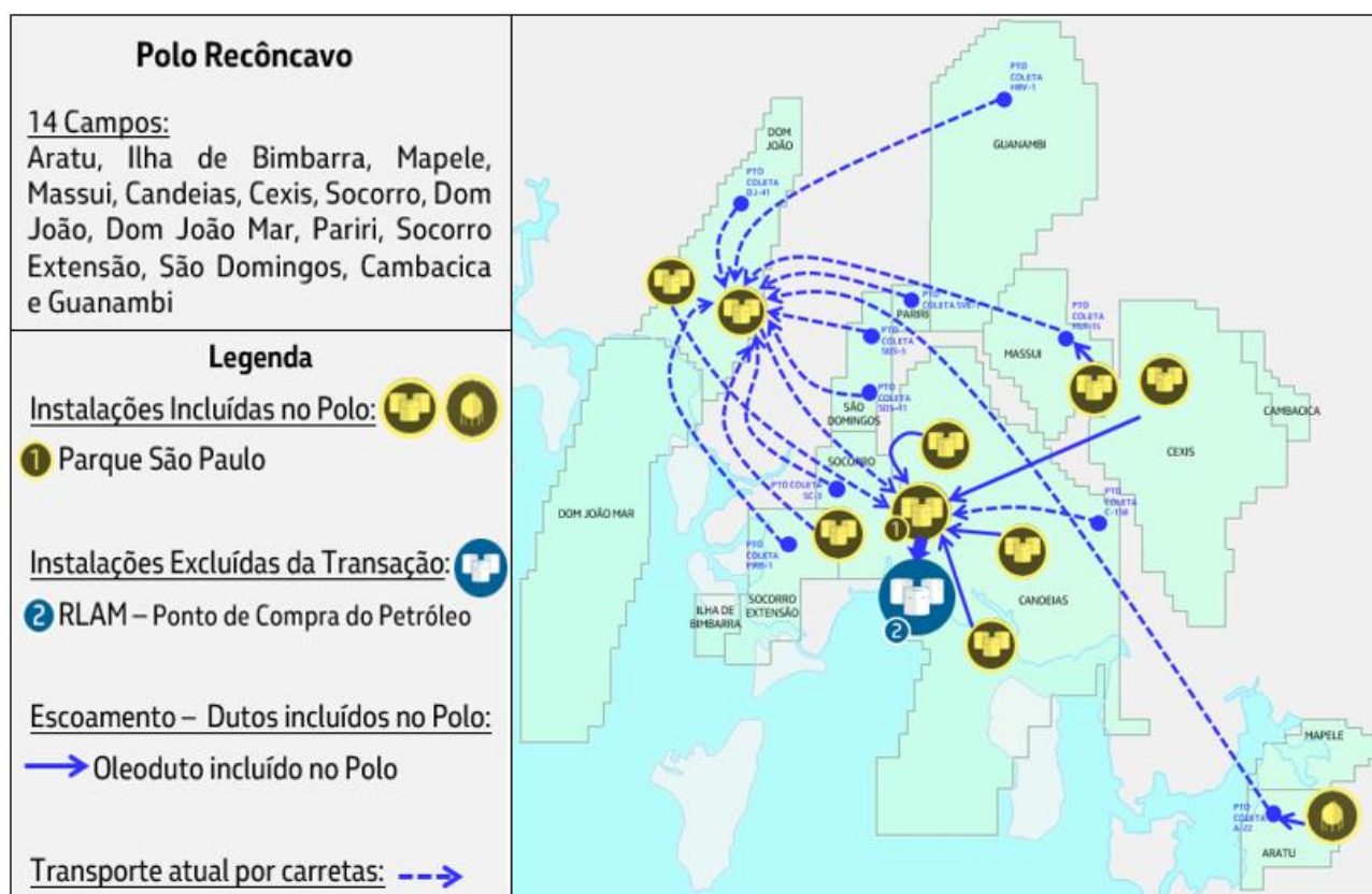
Figura 2 - Fluxo da Produção de Petróleo do Polo Recôncavo
